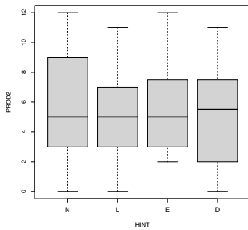
(d) Box-plot for PROD 2
